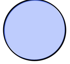
వృత్తం
