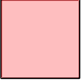
చతురస్రం
