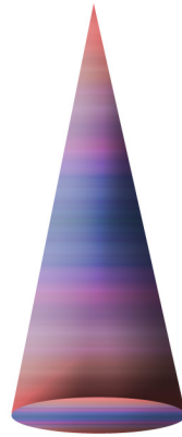
శంఖం
