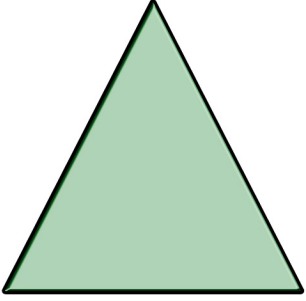
త్రిభుజం
