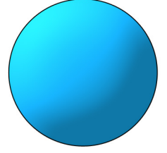
గోళం
