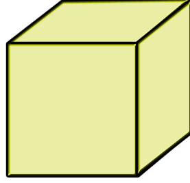
ఘనచతురస్రం
